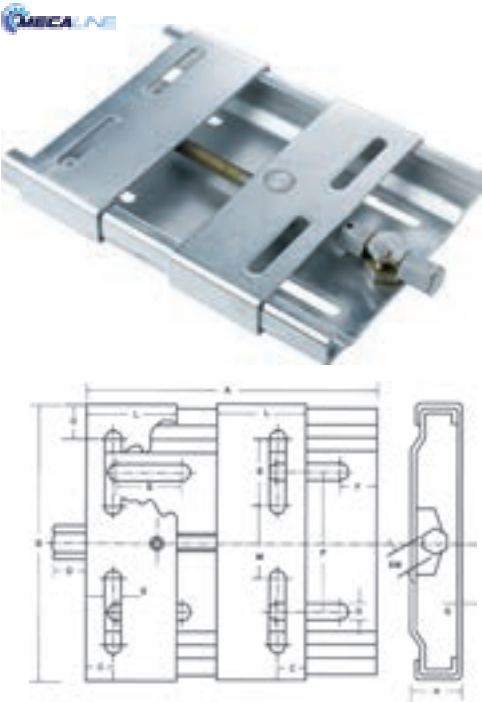
MOTOR BASES GLISSIÈRES MOTEUR BASES DE MOTORES MOTORSPANNSCHIENEN SLITTE PER SCORRIMENTO MOTORE MOTORVOETEN
